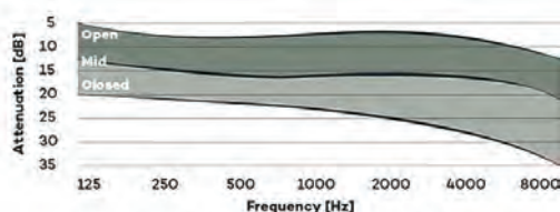
Die vom Hersteller ermittelten Frequenzminderungskurven.
